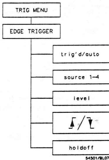
Figure 6-1. Edge Trigger Menu
